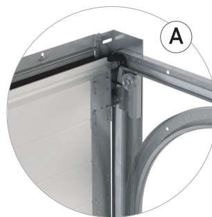
Fig. 1. Dragfjäder placerade horisontellt i frontskenan
